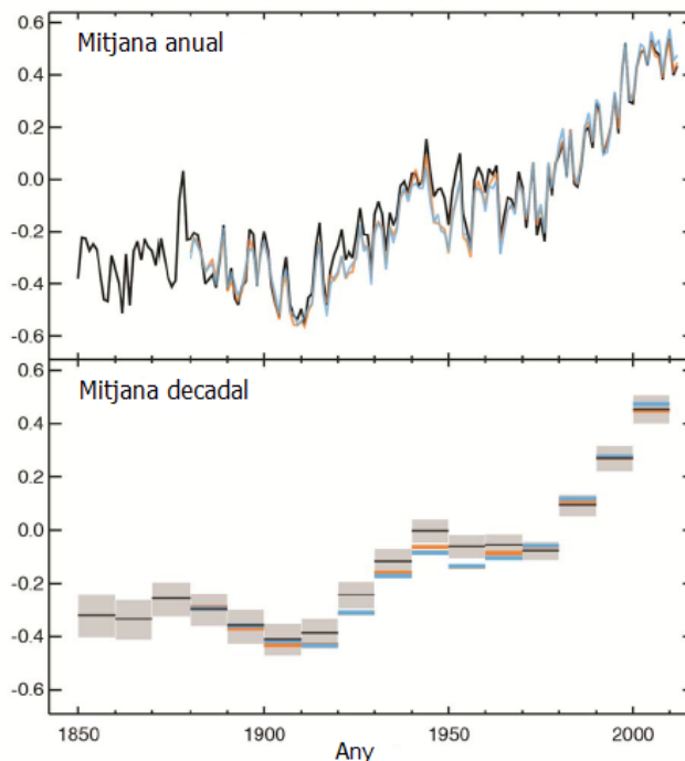
Gràfic 1. Anomalies observades de la temperatura mitjana global, des de 1850 a 2012. A la part de dalt, mitjanes anuals; a la part de baix, mitjanes per dècada. Les anomalies es refereixen a les temperatures mitjanes del període 1961-1990.
