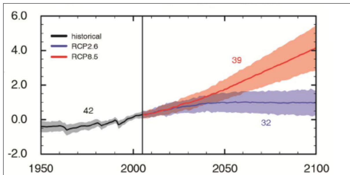
Gràfic 2. Simulacions de l'evolució de la temperatura mitjana global anual de 1950 a 2100, en relació al període 1986-2005. En negre hi ha l'evolució històrica simulada del clima passat, mentre que les projeccions del clima futur es mostren en color blau per la hipòtesi més optimista i en vermell per la més pessimista. L'ombrejat indica el marge d'incertesa per cadascuna de les projeccions.
